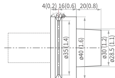
DIN 69893 HSK-E40
