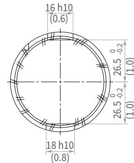
PS-806 (NIKKEN)
