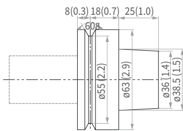
DIN 69893 HSK-F63
